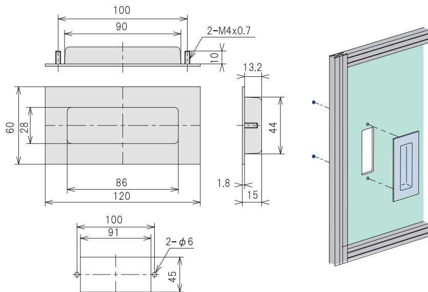
取付加工図
