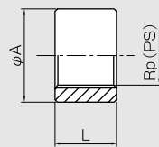
ハーフソケット ストレート (HSS)
