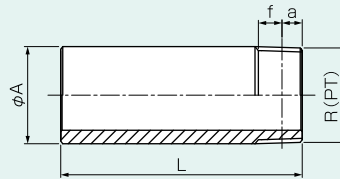
片ねじ
