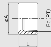
ハーフテーパソケット (HPTS)
