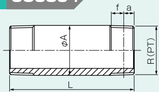
両ねじ
