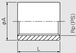
ストレートねじ厚肉 (SJ)
