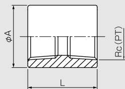
テーパねじ (SPT)
