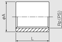
ストレートねじ (S)
