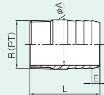
ホースニップル (丸) (CHNI)
