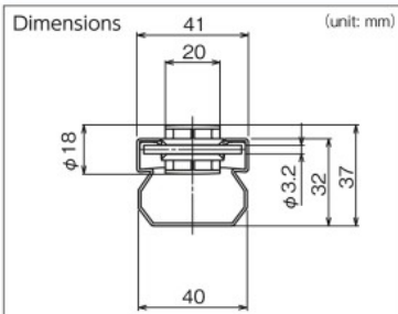
V-1820ECON
