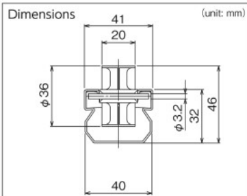
V-3620ECON
