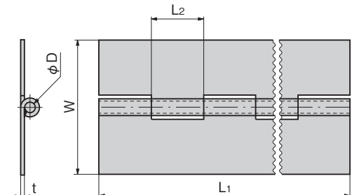
แกนทำจากสแตนเลส Shaft is made of stainless steel
