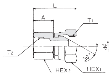
接続口金具 : SR-01・SR-02
