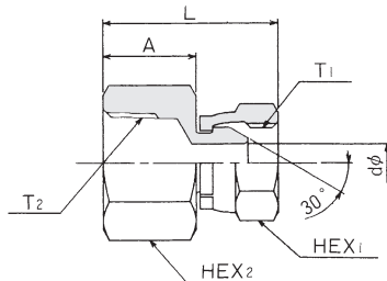
接続口金具 : SR-01・SR-02
