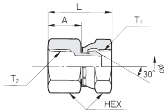
接続口金具 : SR-01・SR-02
