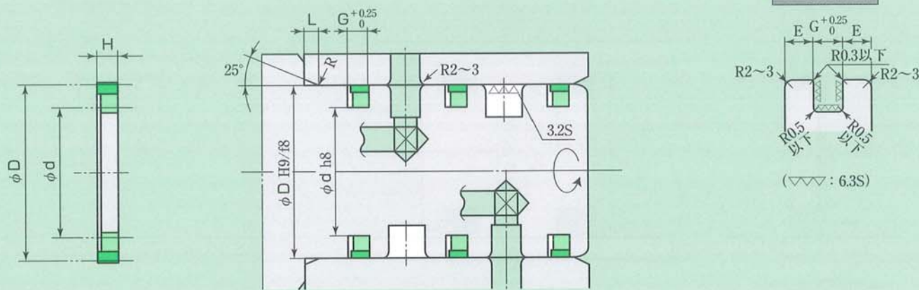
STKシール (STRタイプ) 寸法表
