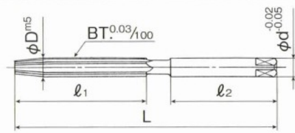
食付き角 1° 1° Chamfer ※図はφ3.0以上の形状です。 Figure is shape of φ3.0 or more
