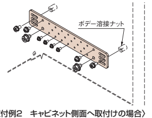
〔取付例2 キャビネット側面へ取付けの場合〕
