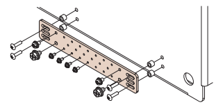
〔取付例：鉄製基板へ取付けの場合〕
