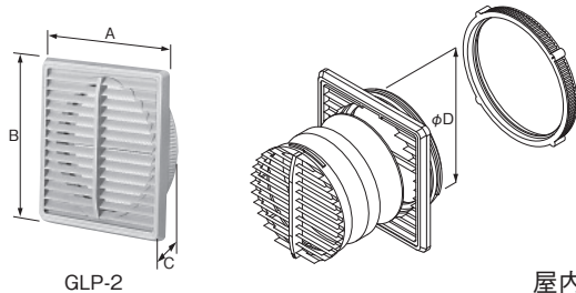
GLP-2
