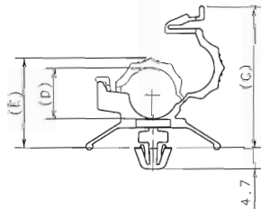
NKSクランプ
