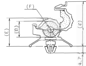
NKSクランプSPタイプ
