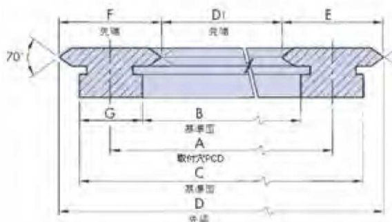
リングレール断面 X-X
