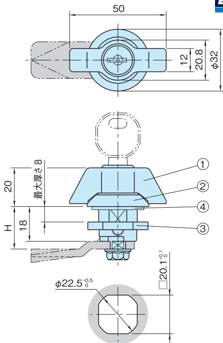
取付穴図
