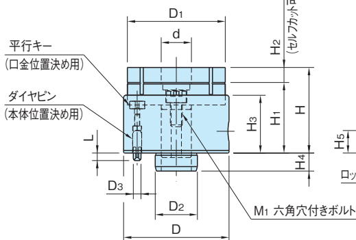
セルフカットワッシャー
